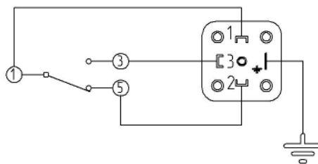
Рисунок 1 – Схема подключения
