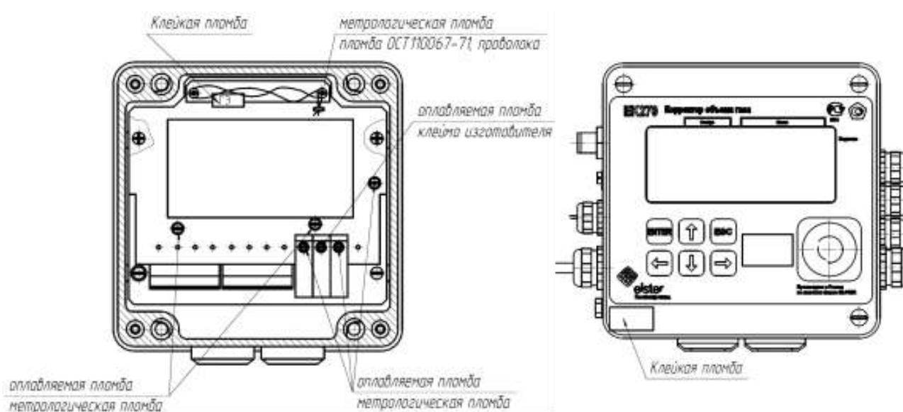
Рис. 3 Расположение пломб
