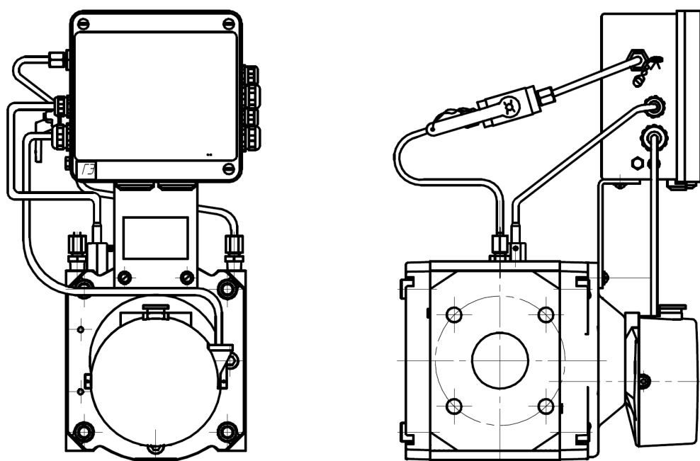
Рисунок 3 Направление потока газа: слева – направо
